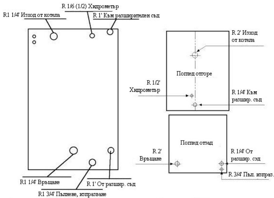
Лънотомат 15-25-40-60 свързване на инсталация
